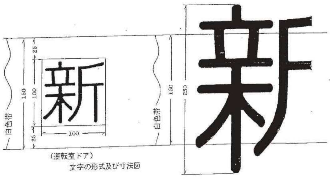
図-3 白色帯と新潟市表示寸法図(エンジン室等)
