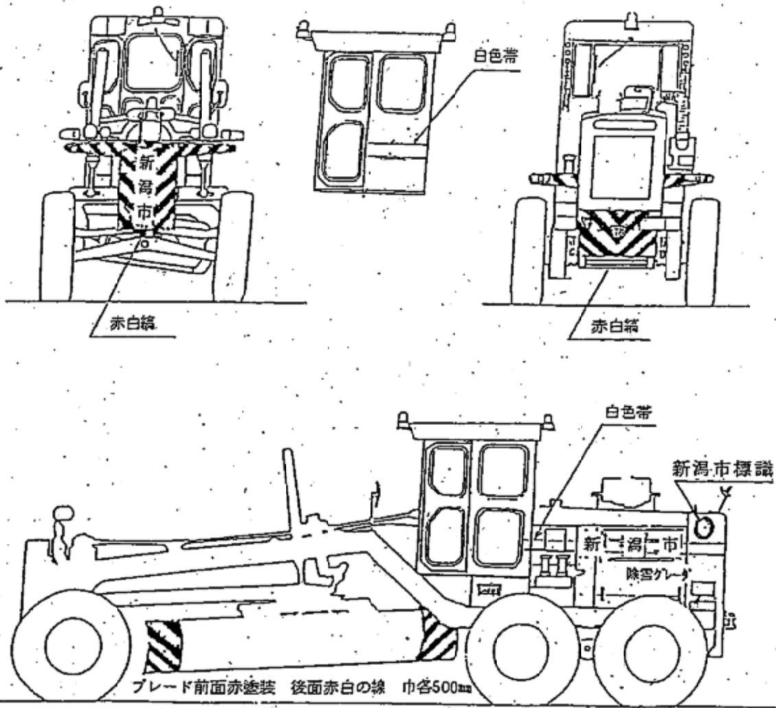
図1 除雪機表示箇所図
