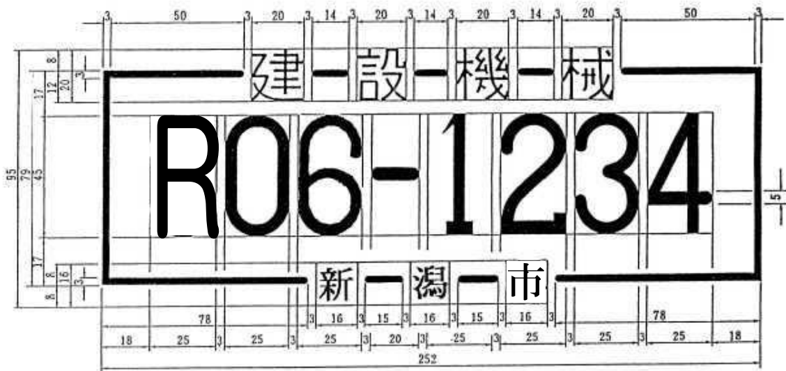
図 4 - 雪寒機械の管理番号寸法図
