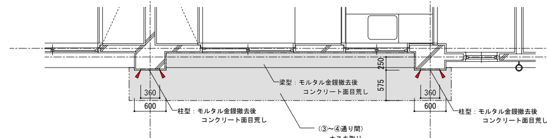
改修前平面図 S=1/50
