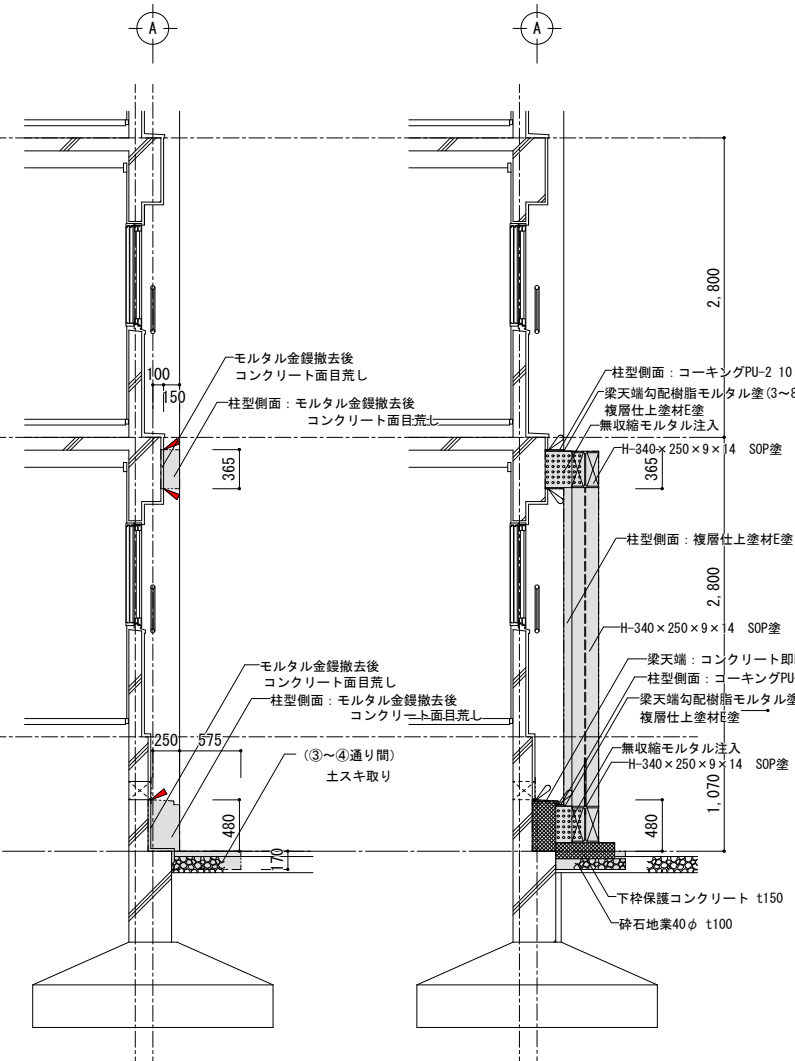
改修前断面図 S=1/50
