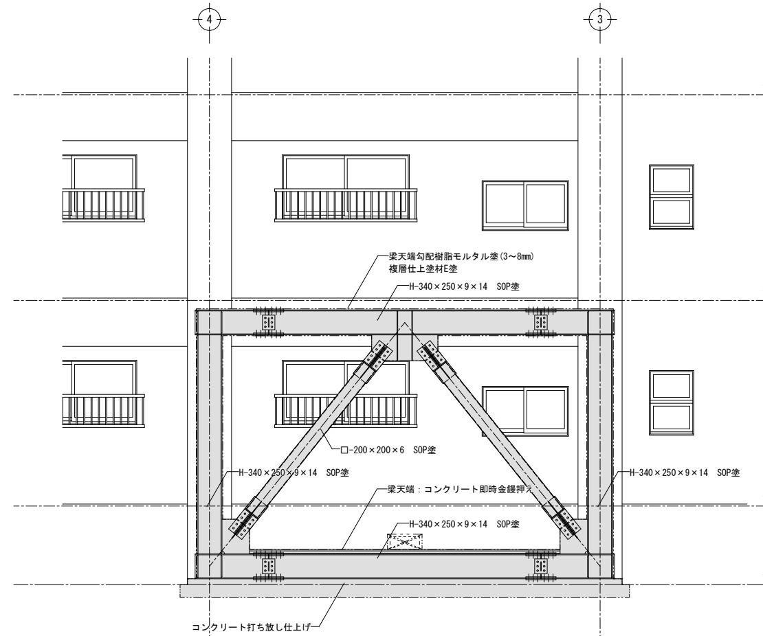
改修後立面図 S=1/50
