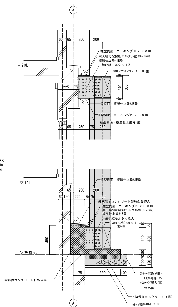
部分断面詳細図 S=1/20
