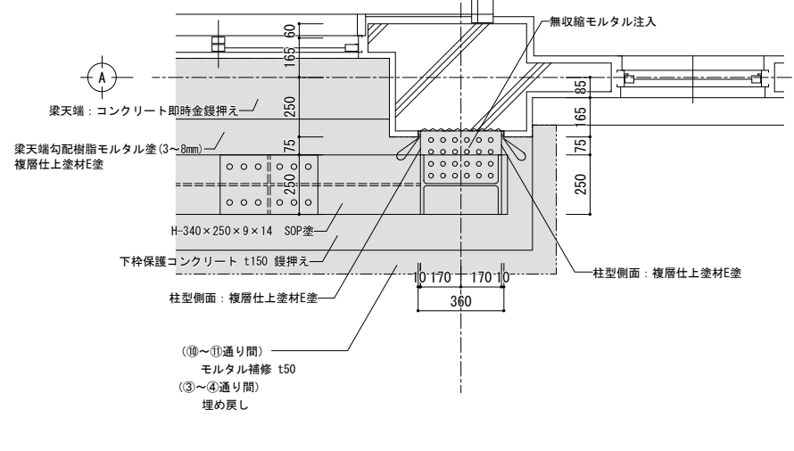
部分平面詳細図 S=1/20
