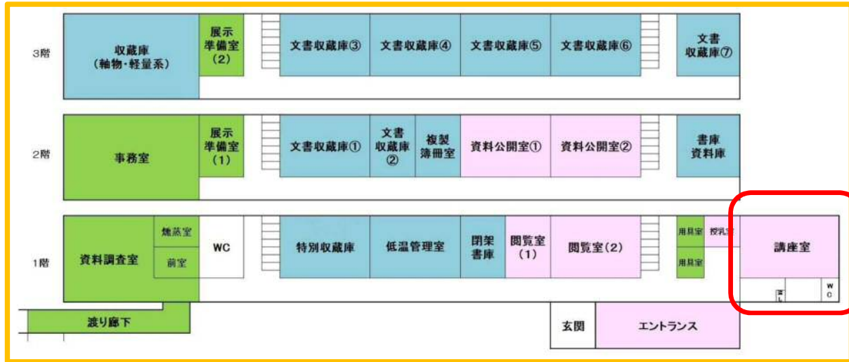
文書館 レイアウト予定図
