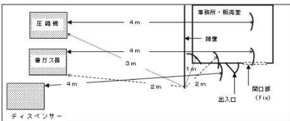
4m未満に建築物の出入口、開口部がある例
