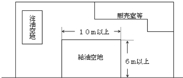
※ 給油空地及び灯油用注油空地の例
