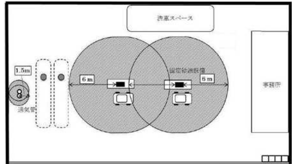
第 14-4 図 給油取扱所の急速充電設備を設置できない範囲例（平面図）
