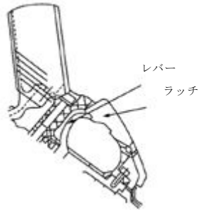
【ノズルレバーがラッチに掛かったまま脱落】
