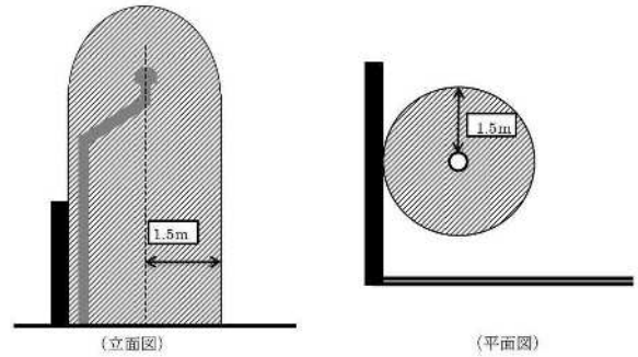
第 14-3 図 通気管の周囲の急速充電設備を設置できない範囲
