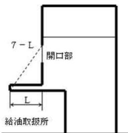
延焼防止上有効なひさしの設置例
