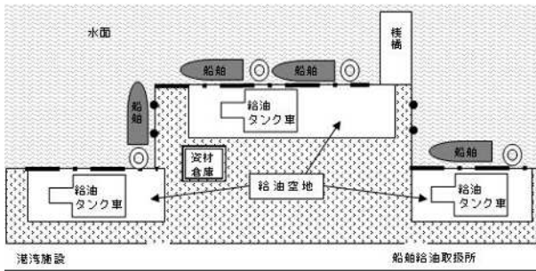
一の船舶給油取扱所内に複数の給油空地を設ける場合の設置例
