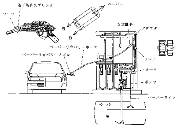
（送油管及び蒸気回収管に取付けられたフロアが給油時に働き、蒸気を回収するもの。）
