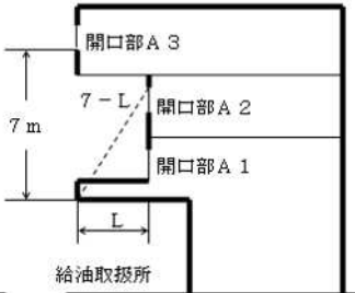
延焼防止上有効なひさしの設置例
