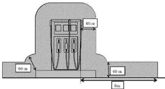
第 14-1 図 固定給油設備（エアギャップがない場合）の周囲の急速充電設備を設置できない範囲
