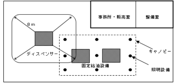
電気設備に耐圧防爆措置が必要な範囲（ディスペンサー外から 8m の範囲内の電気設備が全て対象）
