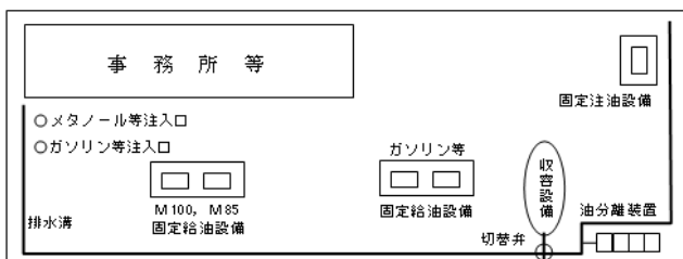
給油空地等の周囲に排水溝等を設ける場合（注入口に係る排水溝等と兼用）の例
