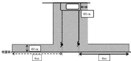
第 14-2 図 懸垂式の固定給油設備の周囲の急速充電設備を設置できない範囲
