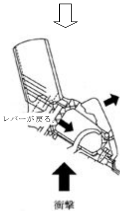
【衝撃でラッチが開放されノズルレバーが戻る】
