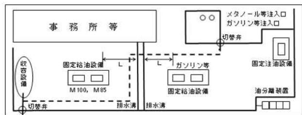
メタノール等の給油空地とガソリン等の給油空地等の周囲にそれぞれ排水溝等を設ける場合（注入口に係る排水溝等と兼用）の例
