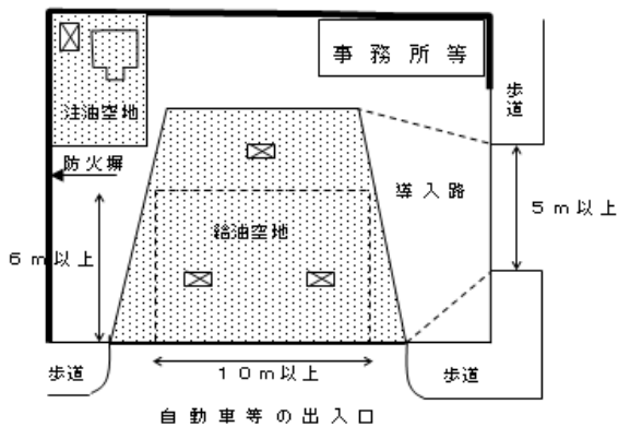
給油空地及び注油空地の例
