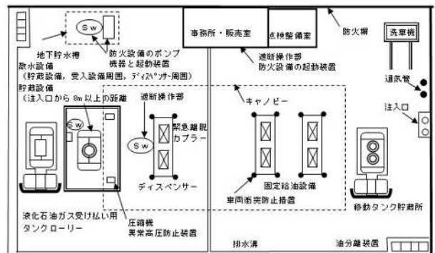
屋外給油取扱所に液化石油ガススタンドを併設した例
