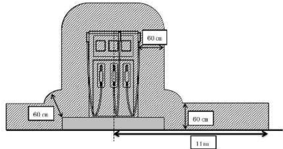
第 14-5 図 固定給油設備（エアギャップがない場合）の周囲の急速充電設備を設置できない範囲
