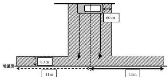
第 14-6 図 懸垂式の固定給油設備の周囲の急速充電設備を設置できない範囲
