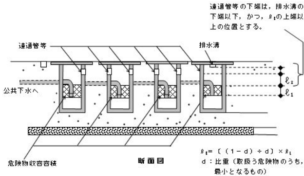
油分離装置の平面図及び断面図
