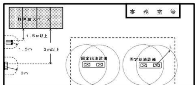
駐停車スペースの例
