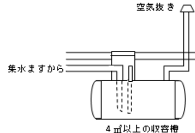
漏えい局限化措置の例
