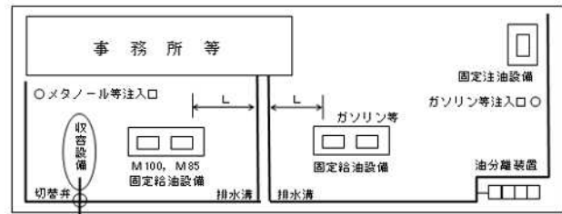
メタノール等の給油空地とガソリン等の給油空地の周囲にそれぞれ排水溝等を設ける場合（注入口に係る排水溝等と兼用）の例
