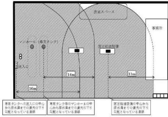
第 14-8 図 給油取扱所の急速充電設備を設置できない範囲例 (平面図)
