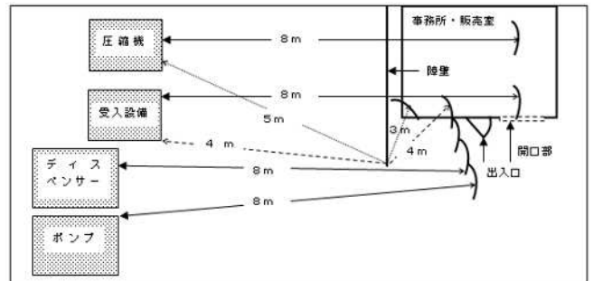
8m 未満に建築物の出入口、開口部がある例
