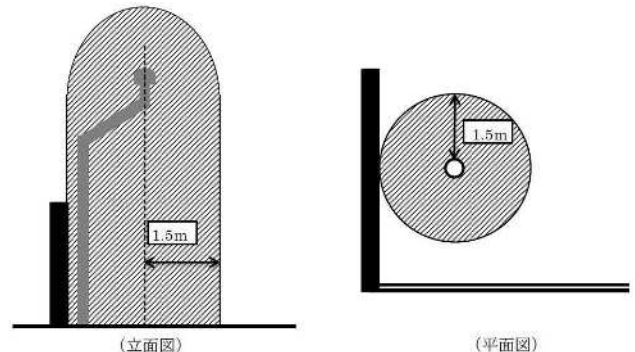
第 14-7 図 通気管の周囲の急速充電設備を設置できない範囲
