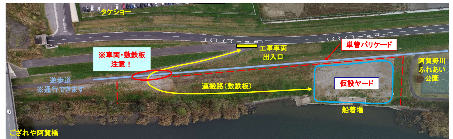
仮設ヤード(阿賀野川ふれあい公園)周辺図
