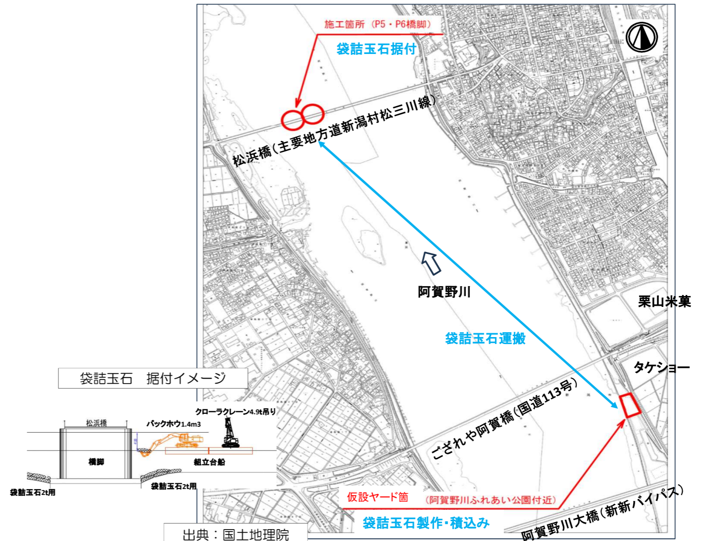
仮設ヤード(阿賀野川ふれあい公園)周辺図
