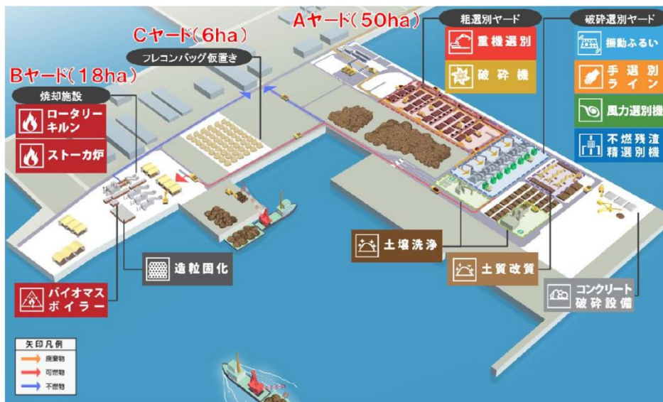
二次仮置場の施設配置例(宮城県石巻ブロック)
