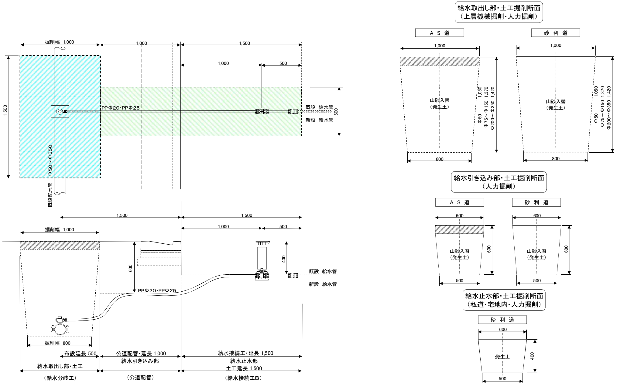
図 - 7 給水接続工B (既設配水管から私有・宅地内の第1止水栓付近までの給水接続に適用)
