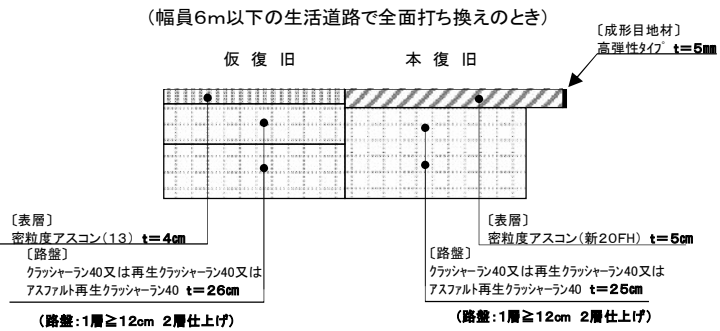
AS道 市道C断面
