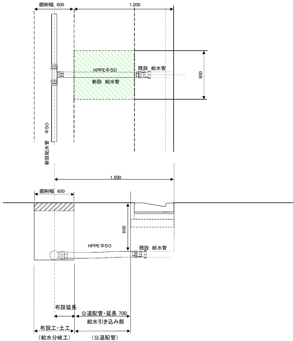
図 - 16 給水接続工C (新設配水管Φ50からΦ50をチーズ分岐して既設配水管Φ50と道路部で給水接続する場合に適用)
