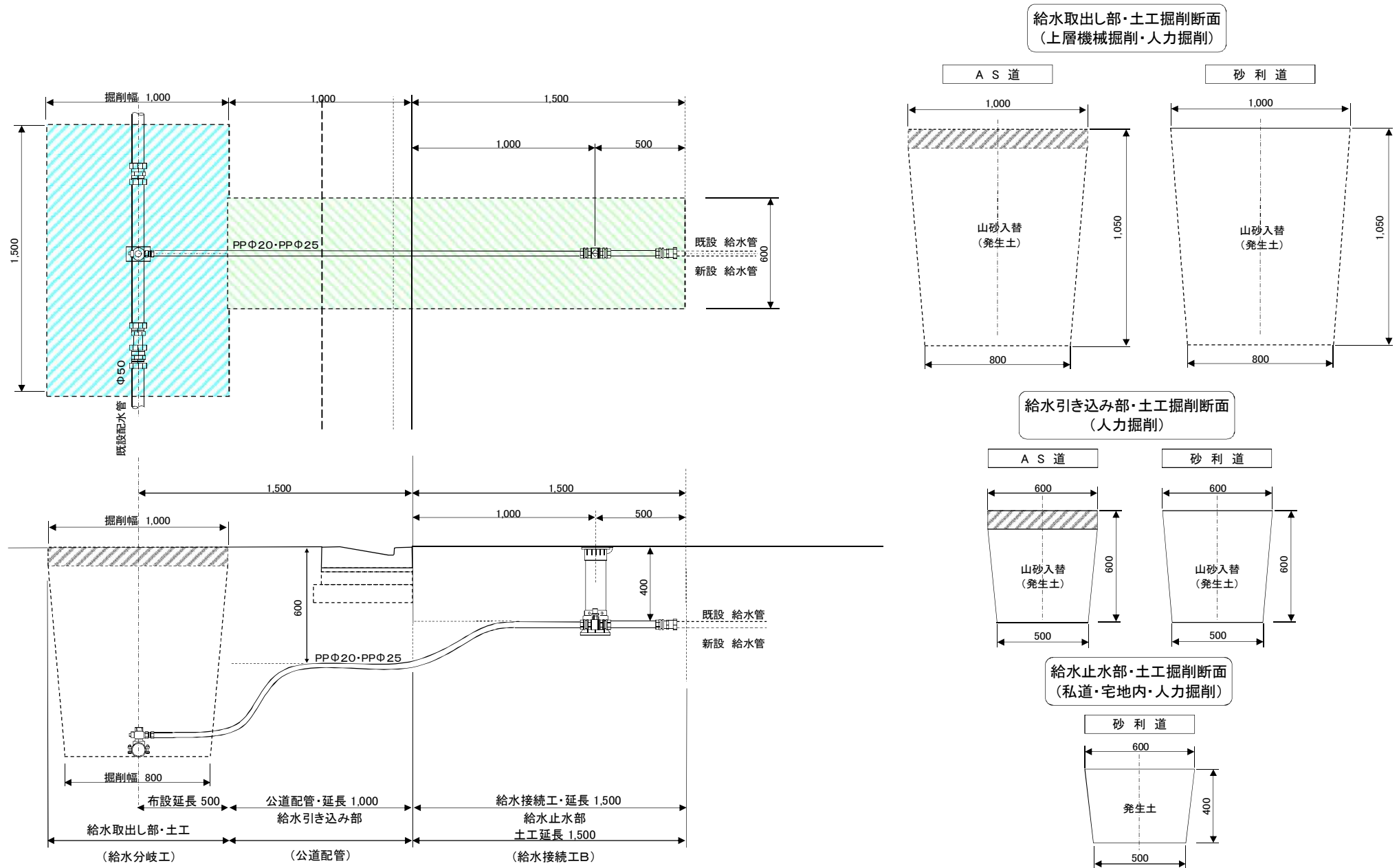
図-9 給水接続工B (既設配水管Φ50を切り落しサドル分岐して私有・宅地内の第1止水栓付近までの給水接続に適用)
