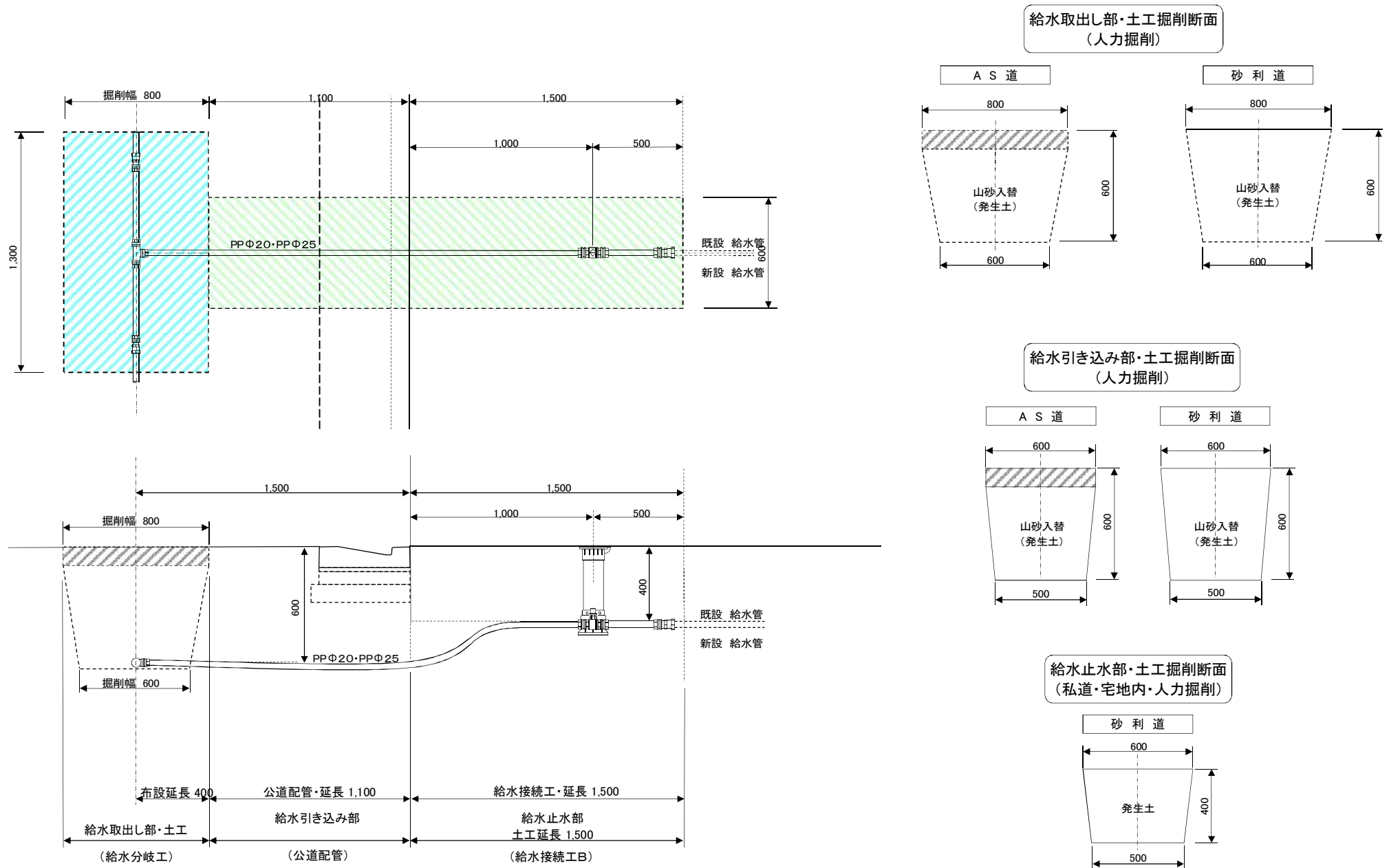
図 - 11 給水接続工B (既設Φ25から切り落としチーズ分岐して私道・宅地内の第1止水栓付近までの給水接続に適用)
