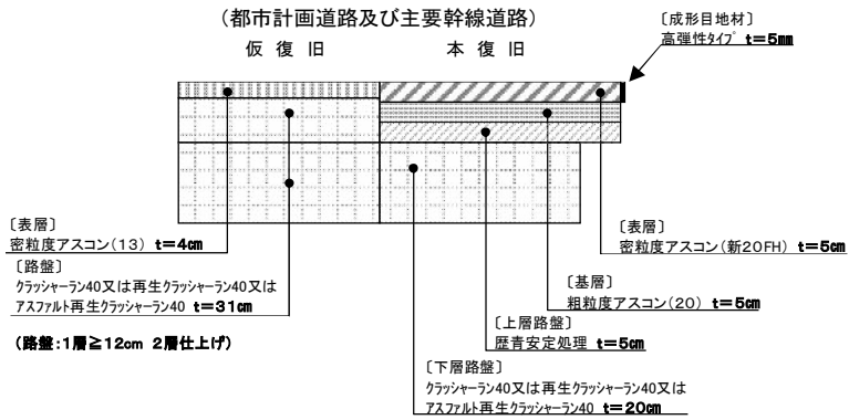
AS道 市道A断面
