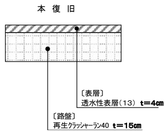
AS道 市道・歩道・透水性舗装
