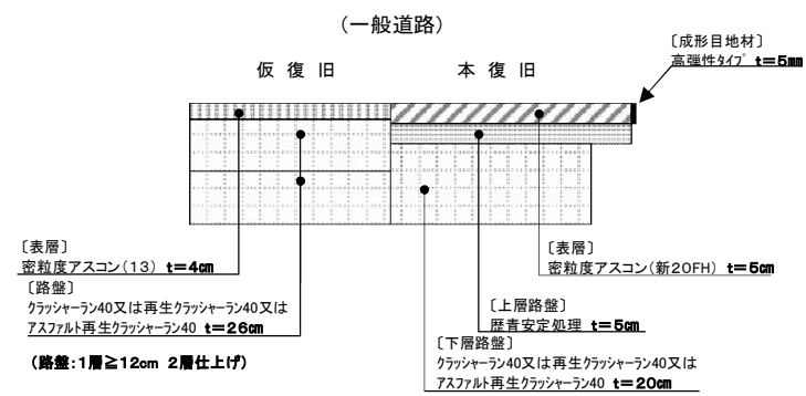
AS道 市道B断面
