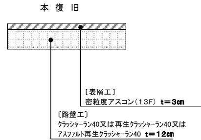
AS道 私道(幅員2m程度)
