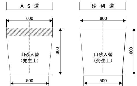
給水引き込み部・給水止水部 土工掘削断面 (人力掘削)
