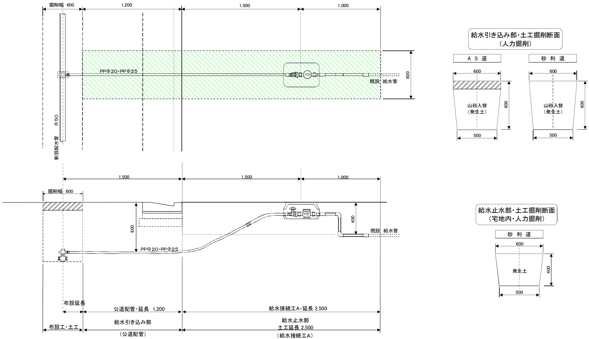
図 - 5 給水接続工A (新設配水管Φ50mmから宅地内メータまでの給水接続に適用)
