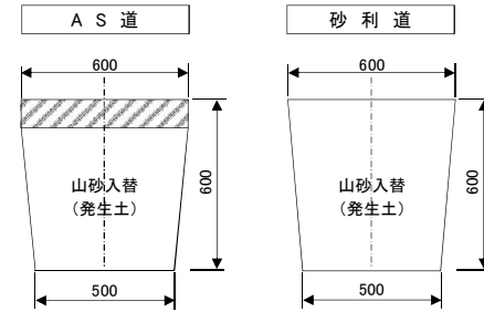
給水止水部・土工掘削断面 （宅地内・人力掘削）
