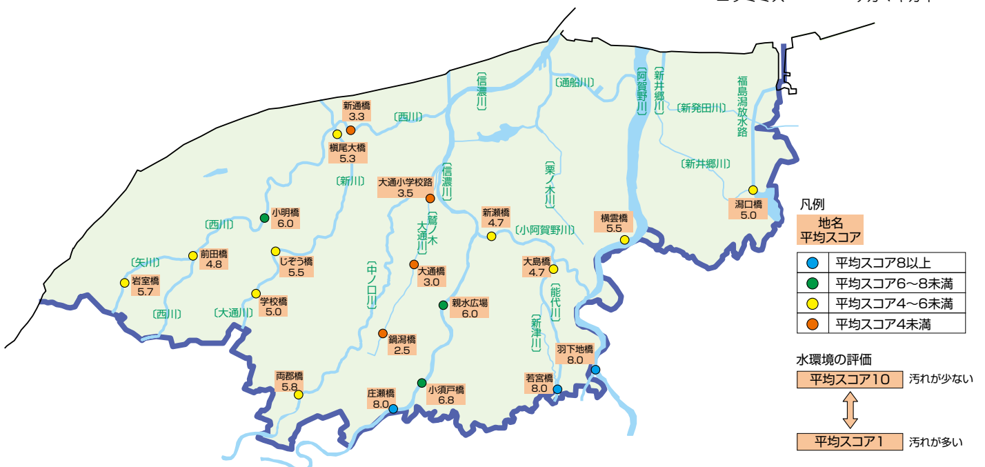
■図-27 スコア法による市内河川の水質状況（平成20～28年）新潟市衛生環境研究所の調査による
