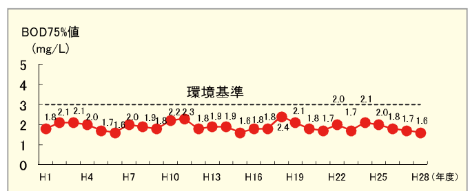
■図-11 福島潟(潟口橋)のBODの経年変化
