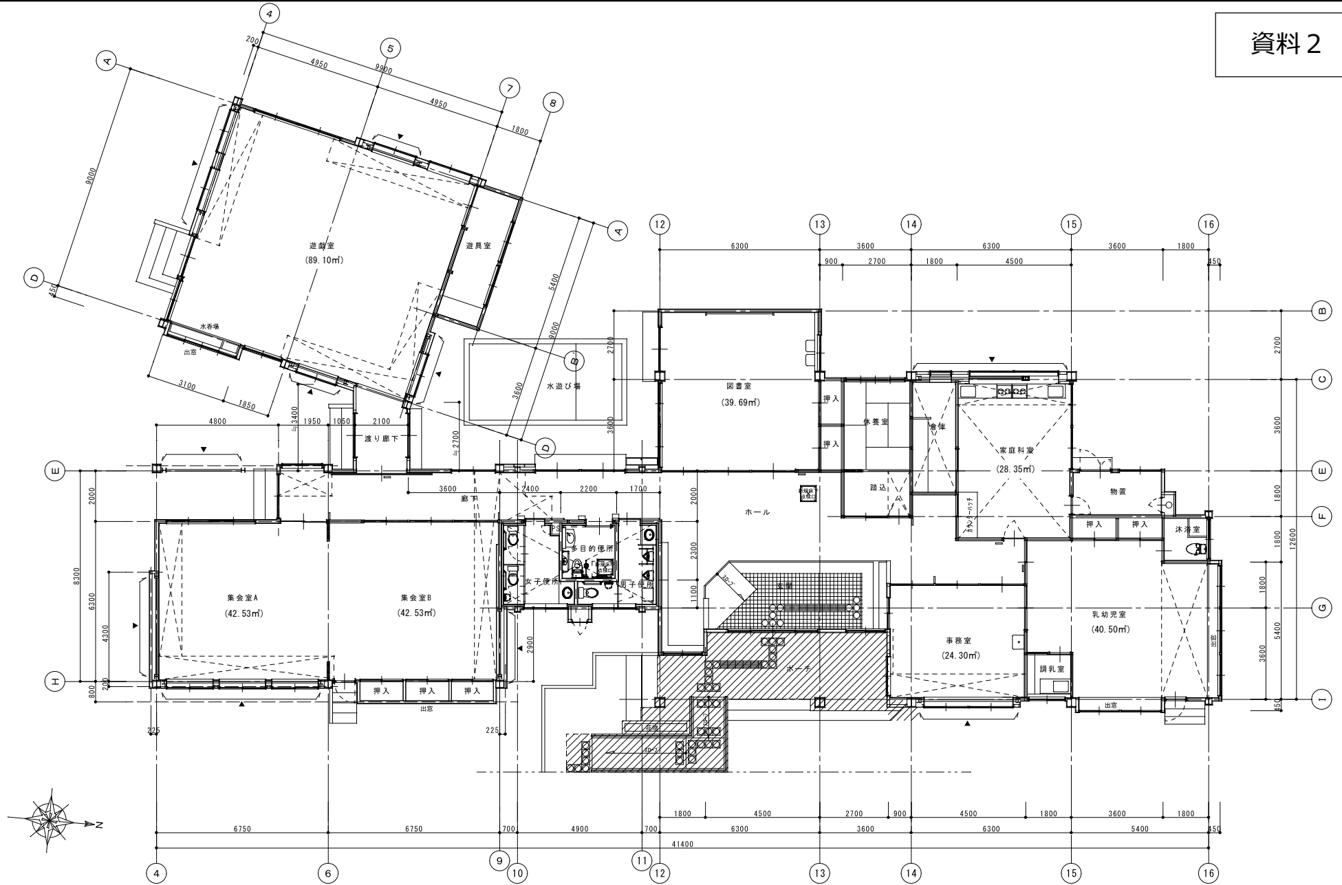
平面図 S=1/100
