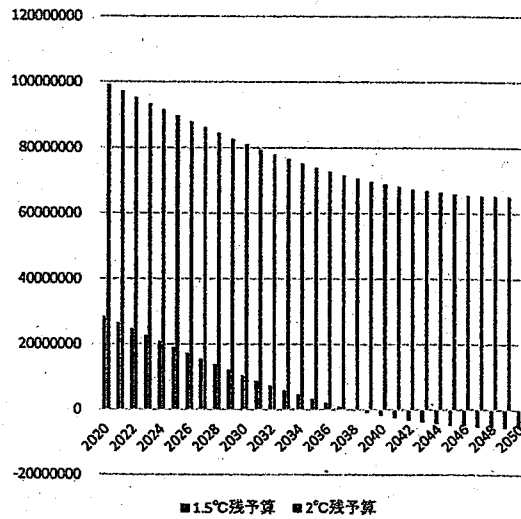
残炭素予算
