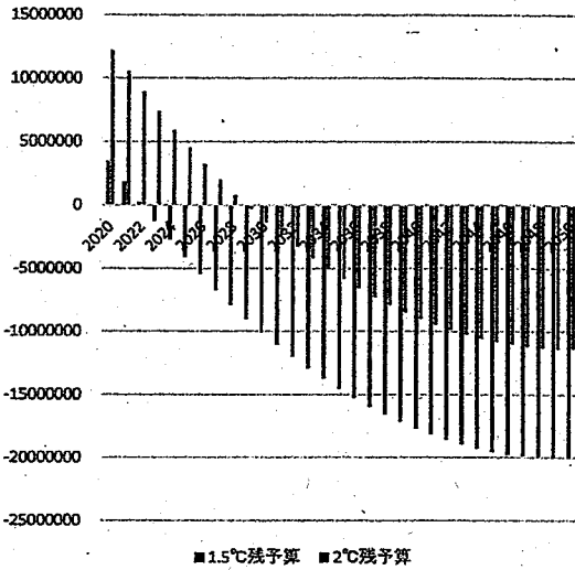
残炭素予算
