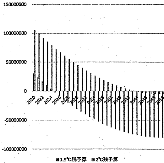
残炭素予算
